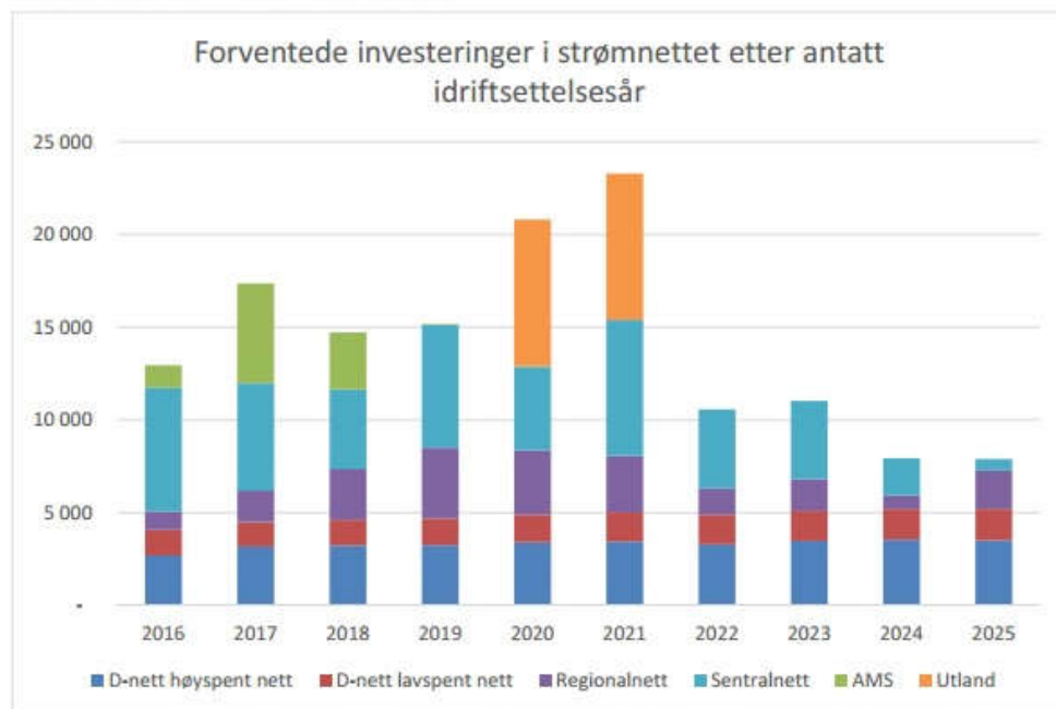
Figur 22 Totale investeringskostnader i Norges strømnnett etter idriftsettelsesår.
